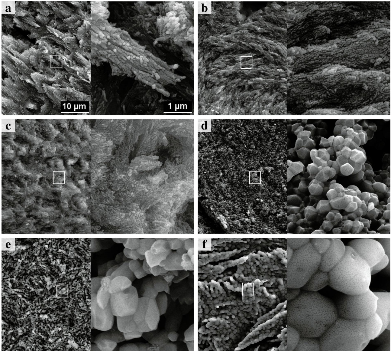
Figura 6 - Fotografias registradas por MEV, com ampliação de 10k e 50kx das amostras: (a) Osso fresco; (b) Queimado a 300 °C; (c) 500 °C; (d) 700 °C; (e) 800 °C; e (f) 1100 °C
