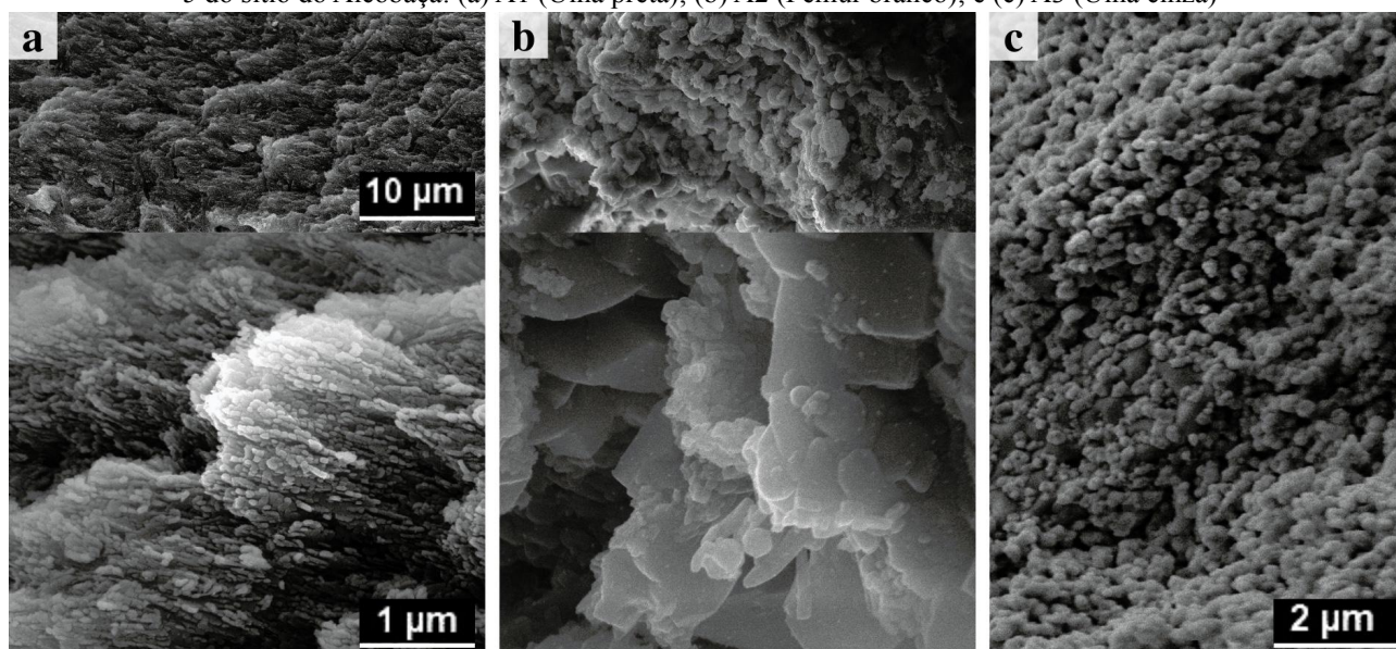
Figura 8 - Fotografias registradas por MEV, com ampliação de 10k e 50k x, das amostras arqueológicas do enterramento 5 do sítio do Alcobaca: (a) A1 (Ulna preta); (b) A2 (Fêmur branco); e (c) A3 (Ulna cinza)
