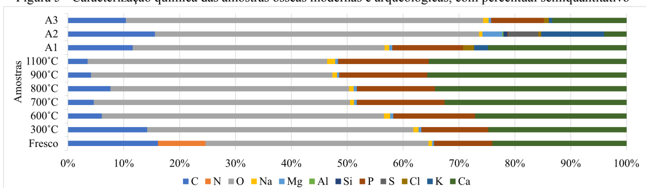
Figura 5 - Caracterização química das amostras ósseas modernas e arqueológicas, com percentual semiquantitativo
